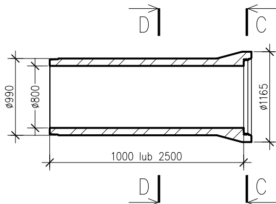
PRZEKRÓJ E-E
